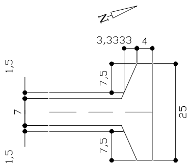
Detalhe cul de sac Esc. Sem escala.
